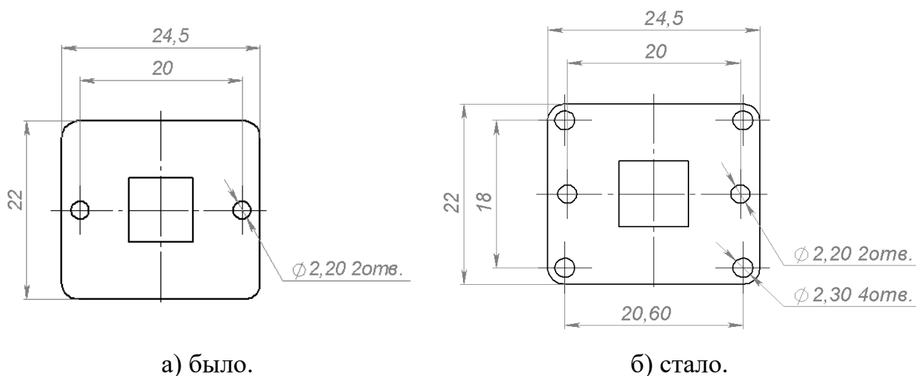
Рисунок 1. Крепёжные отверстия модулей.
